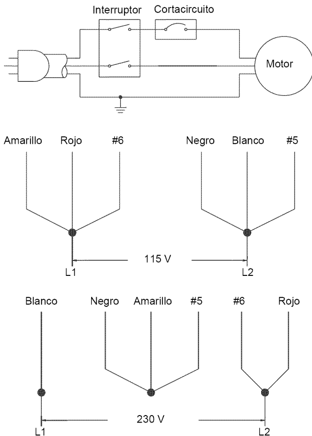
Figura 5 – Diagrama del Cableado
