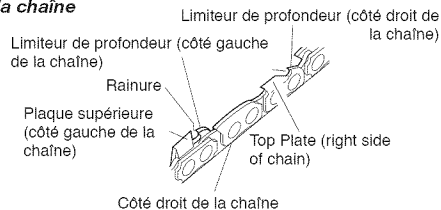
Figure 15 - Emplacement des pièces de la chaîne
