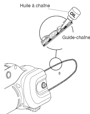
Figure 8 - Huiler la chaîne et le guide-chaîne
