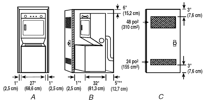
A. Encastrement
