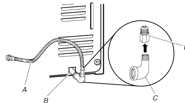
A. Connecteur de gaz souple de 3/8"
