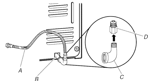
A. Conector flexible de gas de 3/8"
