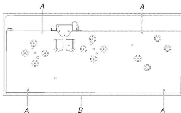
A. Emplacements des trous de montage B. Avant de la table de cuisson
