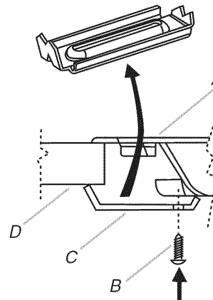
A. Table de cuisson B. Vis de montage C. Bride A D. Plan de travail
