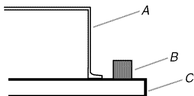
A. Boîte des brûleurs B. Bande de mousse C. Table de cuisson
