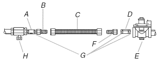
A. Raccord droit de 3/8" B. Raccord d'adaptation de 3/8" C. Raccord flexible D. Raccord droit de 3/8" E. Détendeur F. Raccord d'adaptation de 3/8" G. Appliquer un composé d'étanchéité. H. Robinet d'arrêt manuel
