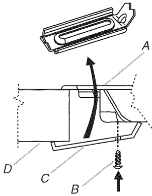
A. Table de cuisson B. Vis de montage C. Bride B D. Plan de travail
