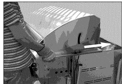
FIG. 09 Une fois le gril sur le chariot, glissez-le vers l'arrière du chariot tel qu'indiqué.
