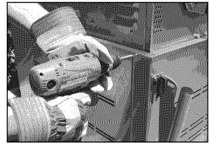
FIG.12 Fixez le gril à la partie arrière du chariot à l'aide de (2) vis phillips fournies (10-24 x 1/2 po).
