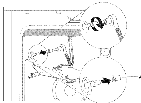
A. Gicleur du brûleur du gril au gaz naturel numéro 52
