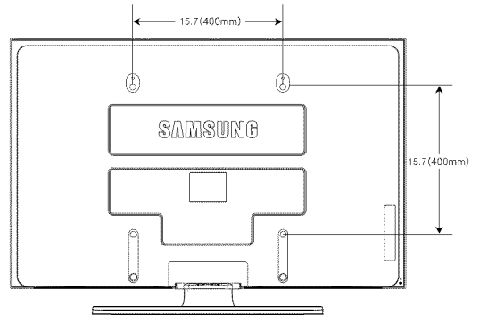
VUE ARRIÈRE
