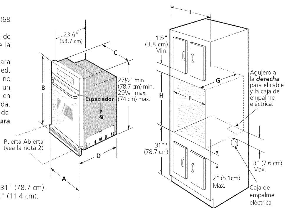
Figura 1- MODELOS CON UN SOLO HORNO (Modelos de horno doble vea la Figura 2)
