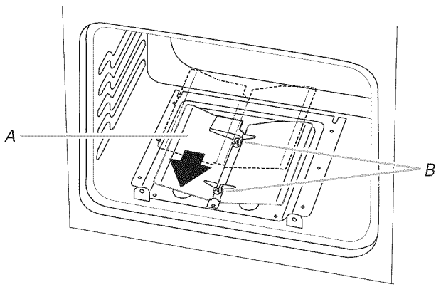
A. Oven baffle B. Wing nuts
