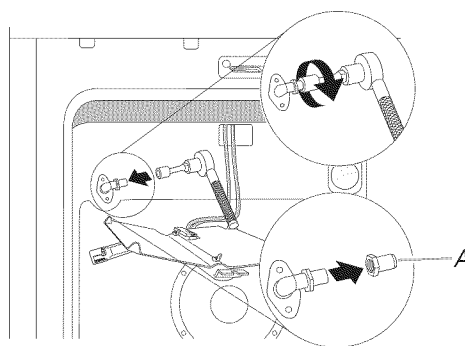
A. Injecteur femelle de 1,42 mm du brûleur du grill pour gaz naturel
