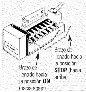
Modelo del Brazo de Llenado
