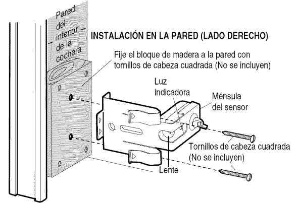
Figure 3 INSTALACIÓN EN LA PARED (LADO DERECHO)
