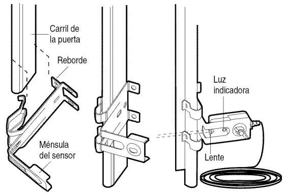
Figure 1 INSTALACIÓN EN EL CARRIL DE LA PUERTA (LADO DERECHO)
