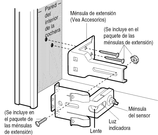
Figure 3 INSTALACIÓN EN LA PARED (LADO DERECHO)
