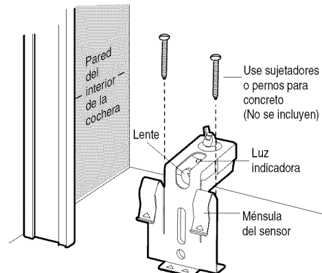
Figure 4 INSTALACIÓN EN EL PISO (LADO DERECHO)
