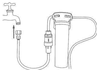
Schéma 3 Fig.5 Raccordement du robinet
