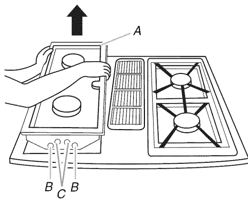
A. Cartouche de brûleur scellé B. Tubes de mixage C. Tiges de l'allumeur
