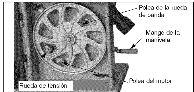
Figura 31 – Cambio de Velocidad de la Hoja
