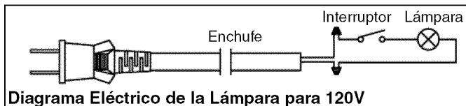
Diagrama Eléctrico de la Lámpara para 120V
