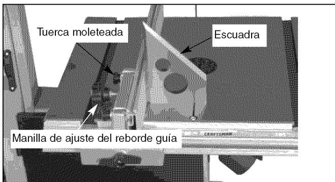
Figura 28 – Ajuste del Reborde
