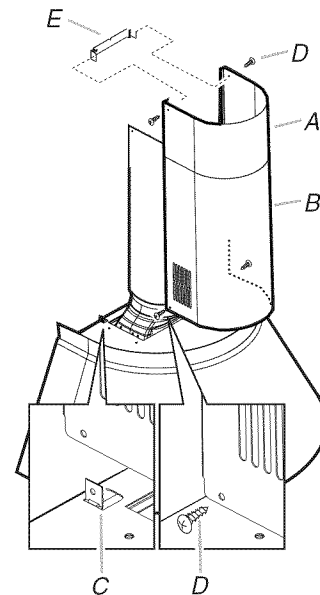
A. Cache-conduit - section supérieure B. Cache-conduit - section inférieure C. Bride de cache-conduit D. Installer les vis de 3 x 9 mm. E. Bride de cache-conduit - section supérieure
