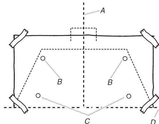
A. Axe central B. Trous pour les vis - emplacements supérieurs C. Trous pour les vis - emplacements inférieurs D. Ligne de référence - hauteur de montage
