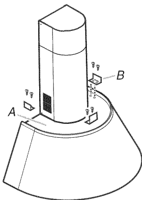
A. Partie supérieure de la hotte B. Supports de garniture
