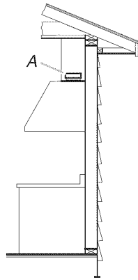
A. Déflecteur
