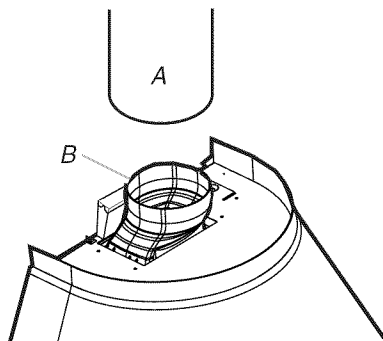
A. Conduit d'évacuation B. Raccord de transition
