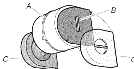
A. Carter du ventilateur B. Manette du filtre C. Filtres à charbon
