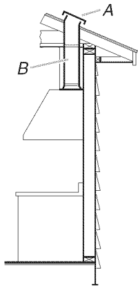
A. Bouche de décharge sur toit B. Conduit dia. 6" (15,2 cm)
