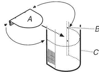
A. Déflecteur B. Trous supérieurs pour les vis C. Cache-conduit - section inférieure
