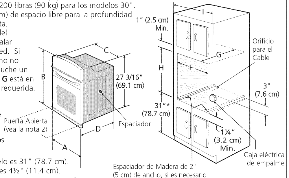
Figura 1 Hornos simples de Pared de 27" y 30" (Para hornos dobles, ver la Figura 2)
