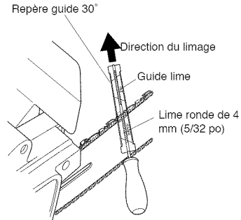
Figure 18 - Position de la lime et du guide lime sur la chaîne
