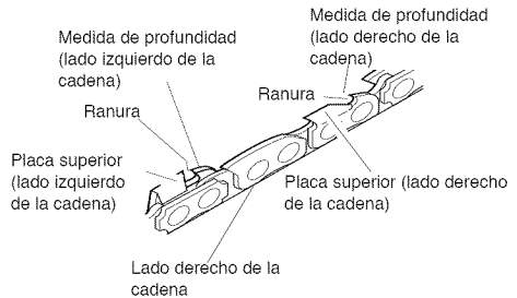
Figura 19 - Posición de las partes de la cadena
