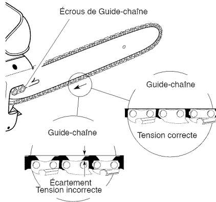
Figure 5 - Réglage de la chaîne
