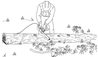
Figura 12 - Trozado del tronco completamente apoyado en el suelo
