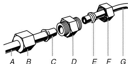
A. Conduit vers le réfrigérateur B. Écrou (fourni) C. Renflement D. Raccord (à acheter) E. Virole (à acheter) F. Écrou (à acheter) G. Canalisations d'eau du domicile
