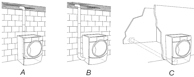
A. Installation d'évacuation standard en décalé par l'arrière B. Installation d'évacuation par le côté gauche ou droit C. Installation d'évacuation par le bas
