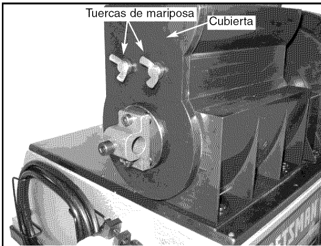
Figura 15 - Retire las tuercas de mariposa y la cubierta.
