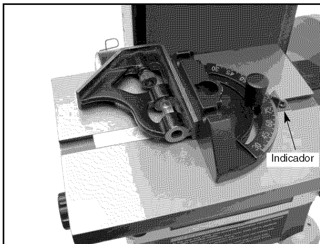
Figura 14 – Ajuste de Cuadratura de la Guía de Ingletes
