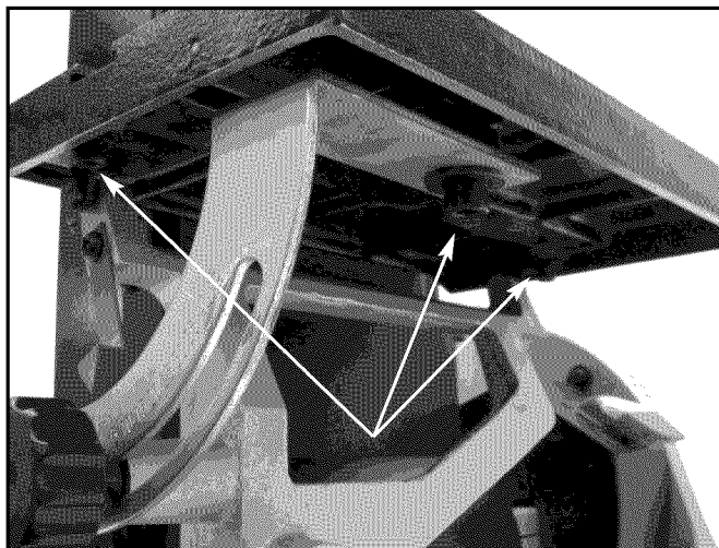
Figura 13 – Ajuste de la Mesa
