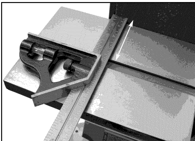
Figura 12 – Verificación del Paralelismo de la Ranura de la Mesa a la Correa
