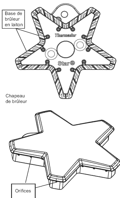
Figure 10 : Éléments de brûleurs Star®
