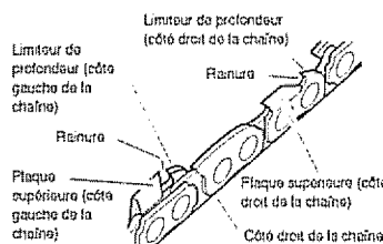
Figure 23 - Emplacement des pièces de la chaîne
