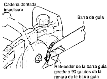
Figura 3 - Bloqueo del retenedor de la barra guía
