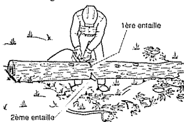
Figure 18 - Tronçonnage d'une bille soutenue aux deux extrémités
