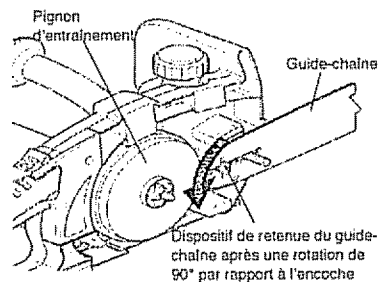
Figure 3 - Verrouillage du dispositif de retenue du guide-chaîne
