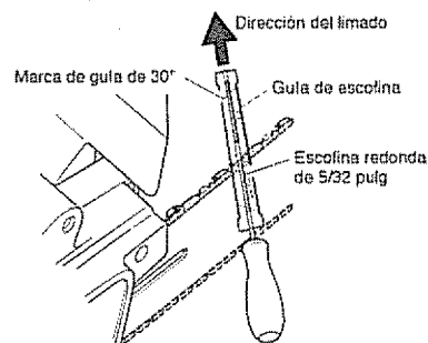
Figura 22 - Colocación de la guía de escofina y de la escofina sobre la cadena
