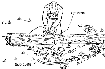
Figura 18 - Trozado del tronco apoyado sobre ambos extremos
