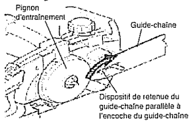
Figure 2 - Déverrouillage du dispositif de retenue du guide-chaîne
