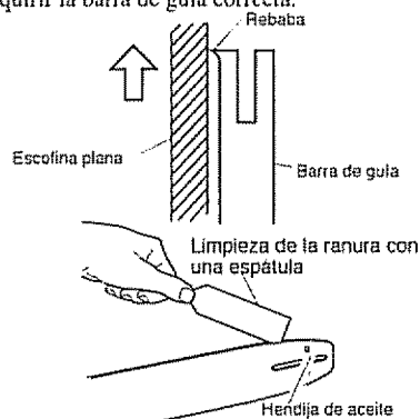
Figura 21 - Mantenimiento de la barra de guía
