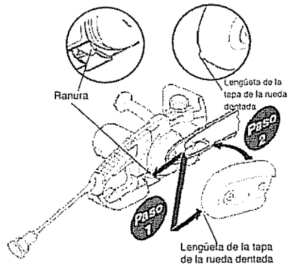
Figura 7- Instalación de la tapa de la rueda dentada
