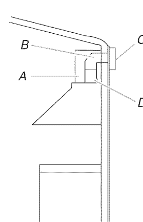
A. Cache-conduit esthétique facultatif B. Conduit dia. 10" (25,4 cm) et coude C. Bouche de décharge murale D. Connexion d'évacuation circulaire de 10" (25,4 cm)
