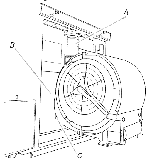
A. Moteur de la tourelle d'aspiration par le bas B. Grande plaque de fermeture C. Ouverture du conduit d'évacuation du ventilateur
