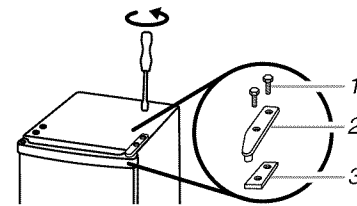
1. Tornillos de \frac{5}{16} pulg. 2. Bisagra superior 3. Calza
