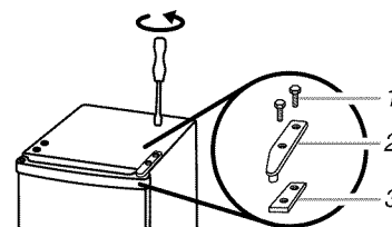
1. Vis de \frac{5}{16} po 2. Charnière supérieure 3. Cale
