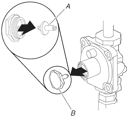
A. Goupille du détendeur B. Capuchon du détendeur
