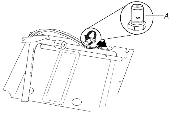
A. Gicleur de gaz naturel (numéro .0723)
