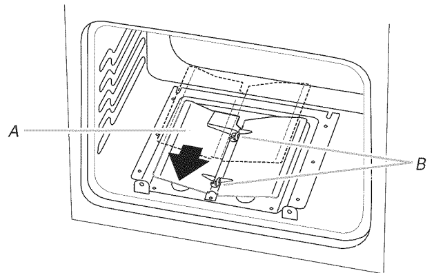
A. Cloison du four B. Wing nuts
