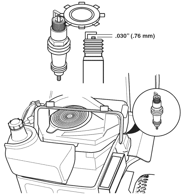
Figure 33. Entrehierro de la Bujía
