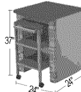
16732-Serving Cart Module
