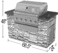
16655 - Barbacoa de Gas
