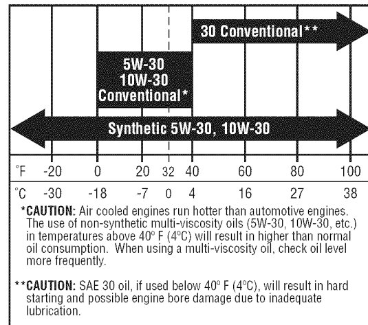
Figura 18. Aceite del motor recomendado
