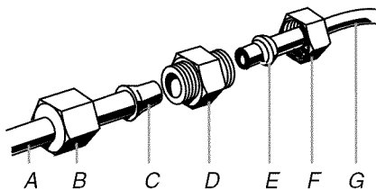
A. Tubería de agua del refrigerador E. Férula (adquirida) B. Tuerca (provista) F. Tuerca (adquirida) C. Bulbo G. Línea de agua de la casa D. Acoplamiento (provisto)
