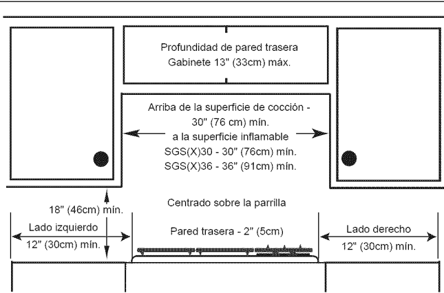
Figura 1: Dimensiones instaladas (desde los bordes de la placa)
