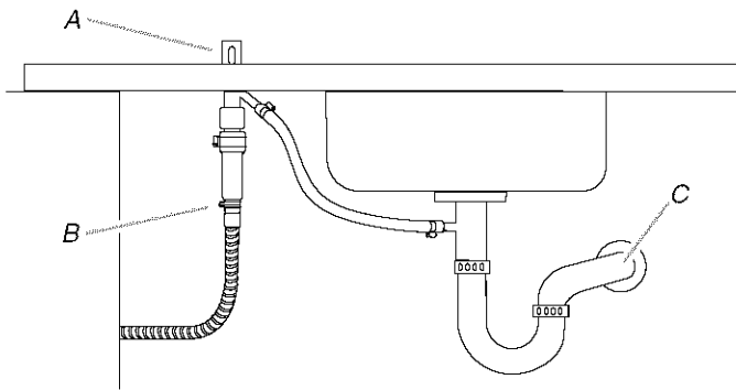
A. Raccord du circuit d'évacuation B. Brise-vidé C. Circuit d'évacuation de la maison
