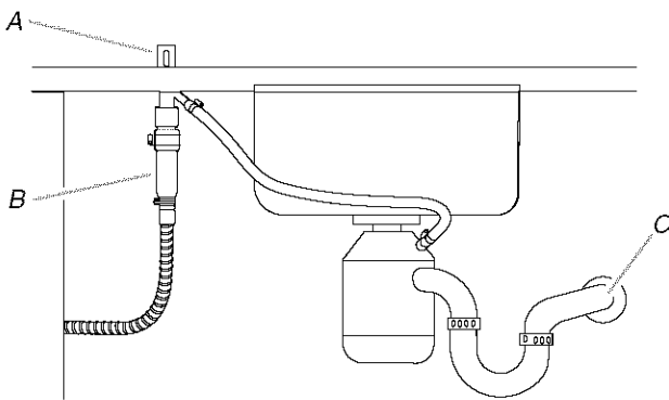
A. Raccord du circuit d'évacuation B. Brise-vidé C. Circuit d'évacuation de la maison
