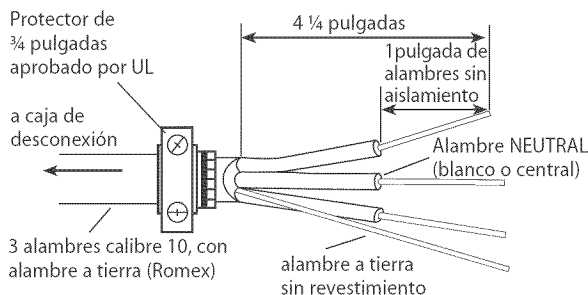
Dibujo 22 Cableado de las conexiones de 4 alambres
