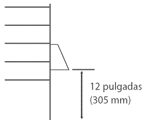
Dibujo 9 Espacio libre del piso a la Campana de extracción
