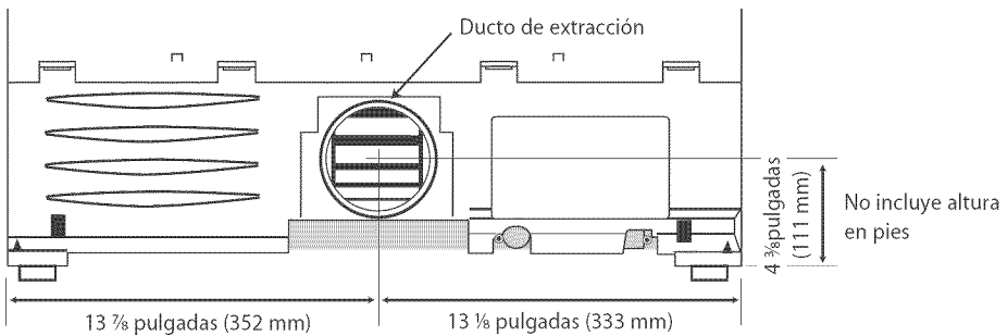
Dibujo 7 Dimensiones del ducto de extracción
