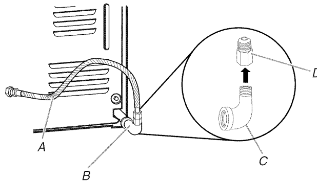
A. Connecteur de gaz souple de 3/8" B. Conduit de la sécheuse de 3/8" C. Coude de conduit de 3/8" à 3/8" D. Adaptateur entre le conduit et le joint conique de 3/8"
