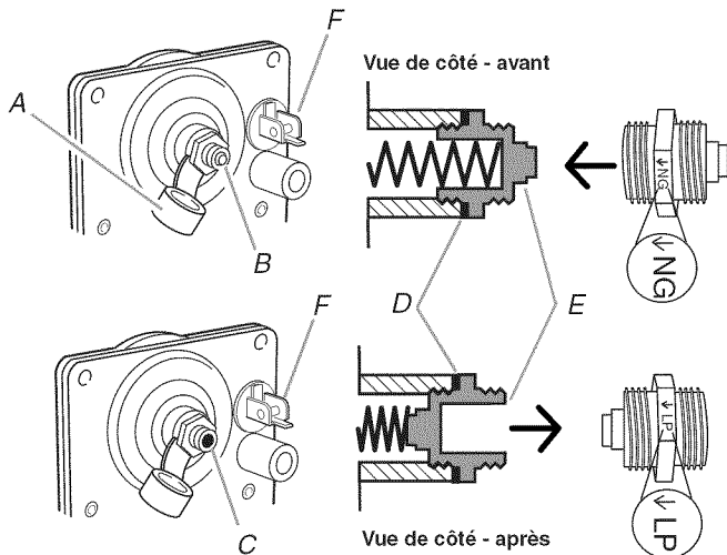
A. Couvercle de plastique B. Capuchon du détendeur; extrémité borgne vers l'extérieur C. Capuchon du détendeur; extrémité ouverte vers l'extérieur D. Joint E. Capuchon du détendeur F. Robinet d'arrêt du détendeur (illustré à la position "ouverte")
