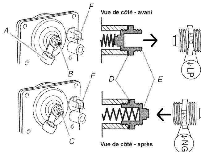
A. Couvercle de plastique B. Capuchon du détendeur; extrémité ouverte vers l'extérieur C. Capuchon du détendeur; extrémité borgne vers l'extérieur D. Joint E. Capuchon du détendeur F. Robinet d'arrêt du détendeur (illustré à la position "ouverte")
