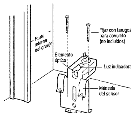
MONTAJE EN PISO (LADO DERECHO)
