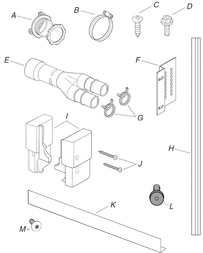
A. Serre-câble \frac{3}{4} " - homologation UL B. Bride de tuyau 1,25" C. 8 vis de bride de montage D. 4 vis de montage de l'appareil E. Raccord Y pour tuyau d'évacuation F. 4 brides de montage G. Brides de tuyau pour tuyau d'évacuation H. 2 bandes de garniture I. Brides pour cornière J. 2 vis - vis de bride pour cornière K. Cornière L. 2 vis de fixation de panneau (certains modèles) M. 10 vis TORX® (certains modèles)
