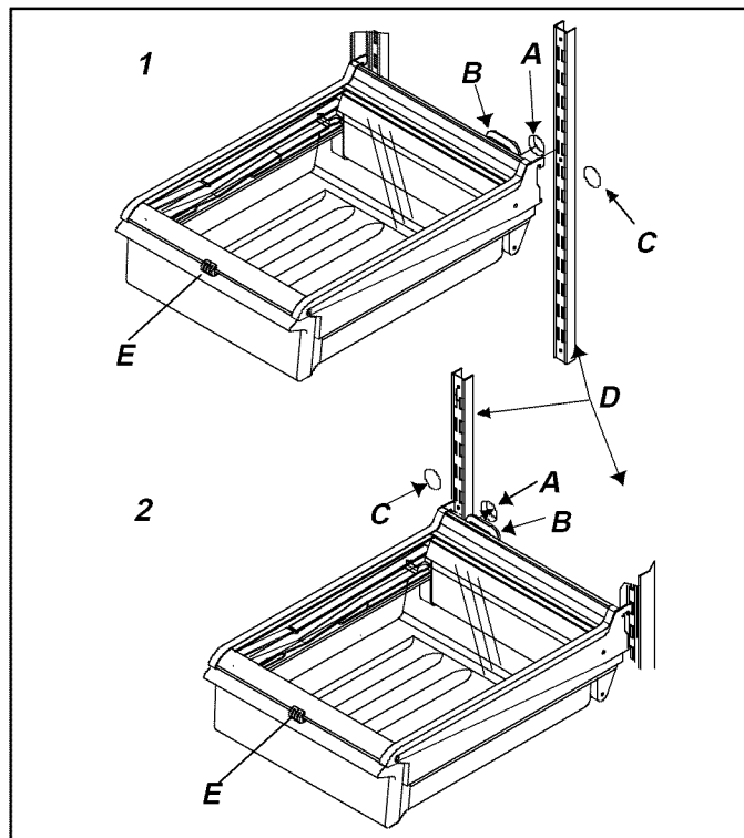
1 Cajón de temperatura controlada instalado en el lado izquierdo del refrigerador.
