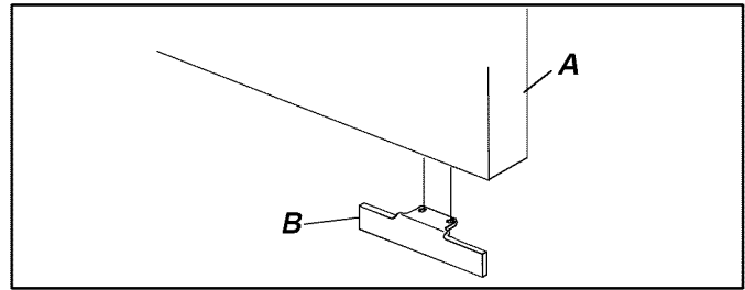
A Porte B Butée de porte
