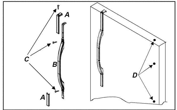
A Adorno del asa B Asa C Tornillos D Tapones
