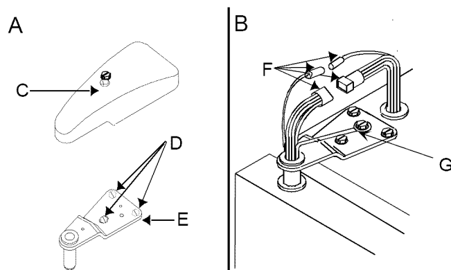
C. Cubierta de la bisagra D. Tornillos de la bisagra de la puerta E. Bisagra superior F. Conectores del alambre G. Alambre a tierra verde
