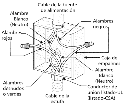
Figura 5 - Sistema eléctrico (ejemplo: caja de empalmes) de 3 alambres (a tierra neutro)
