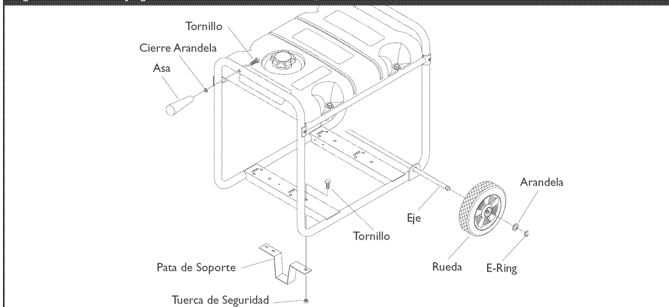
Figura 14 — Instale el Juego de Ruedas
