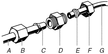
A. Tubería de agua del refrigerador D. Acoplamiento (adquirido) B. Tuerca (provista) E. Fécula (adquirida) C. Bulbo F. Tuerca (adquirida) G. Línea de agua de la casa
