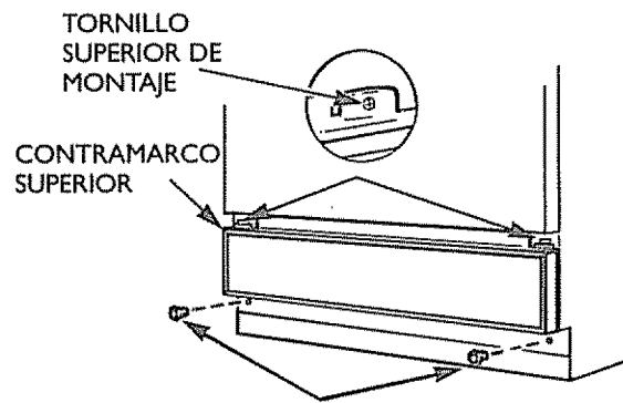
TORNILLOS DE SUJECION DEL PANEL INFERIOR
