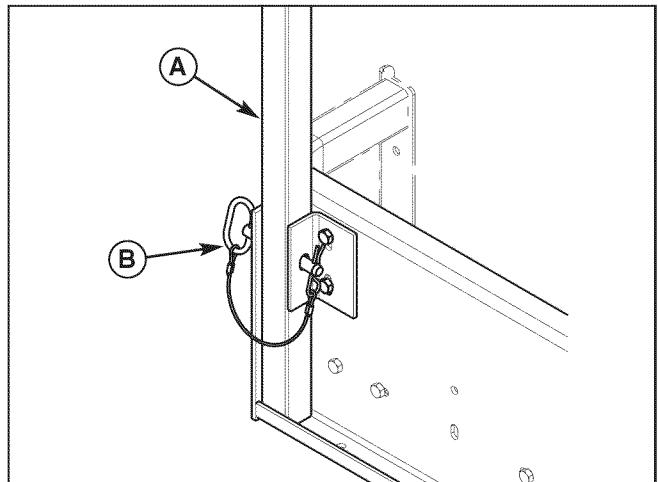
Figura 62. Remoción de los pasadores de enganche
