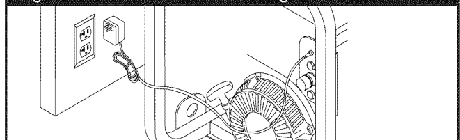
Figura 17 — Enchufe Hembra del Cargador de Flotación
