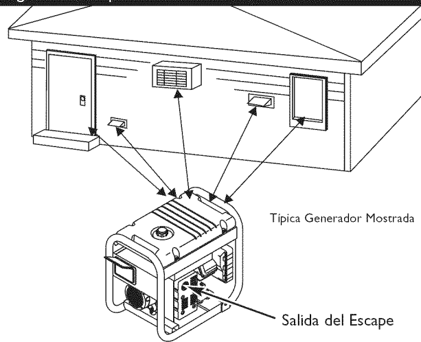
Figura 11 — Espacio Libre Alrededor del Generador
