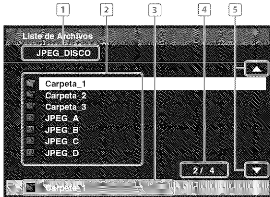
Ej.) JPEG
