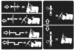
RUEDA LIBRE (Solamente para los modelos automaticos)
